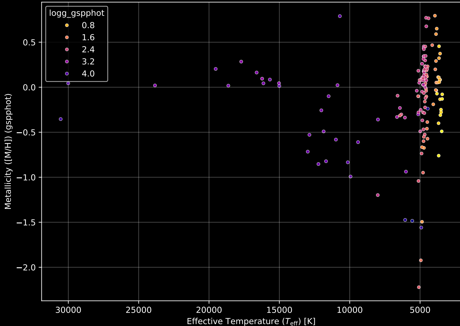
APOGEE DR17 Field: [018-02] Stellar Population Parameters (n= 144)
